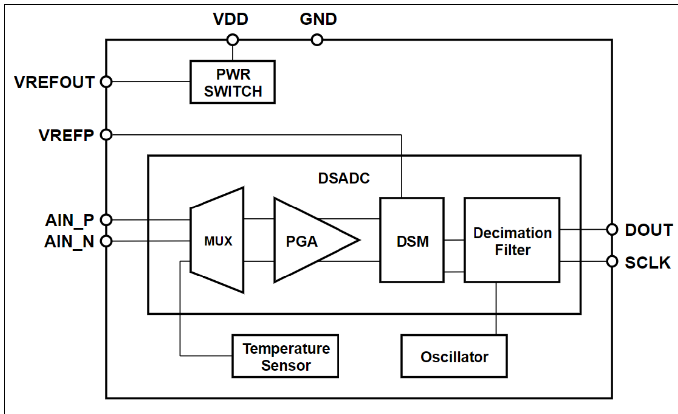
图 1: PMD040B 图框
